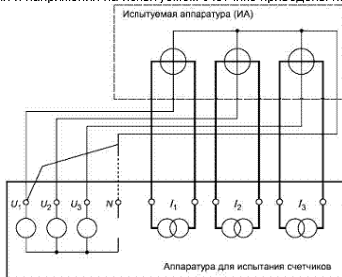
Рисунок С.1 - Схема моделирования состояния замыкания на землю в фазе 1
