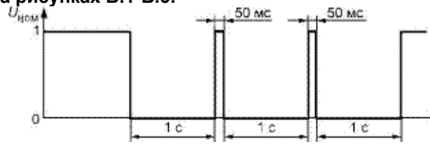
Рисунок В.1 - Прерывания напряжения \Delta U = 100\% , продолжительность 1 с
