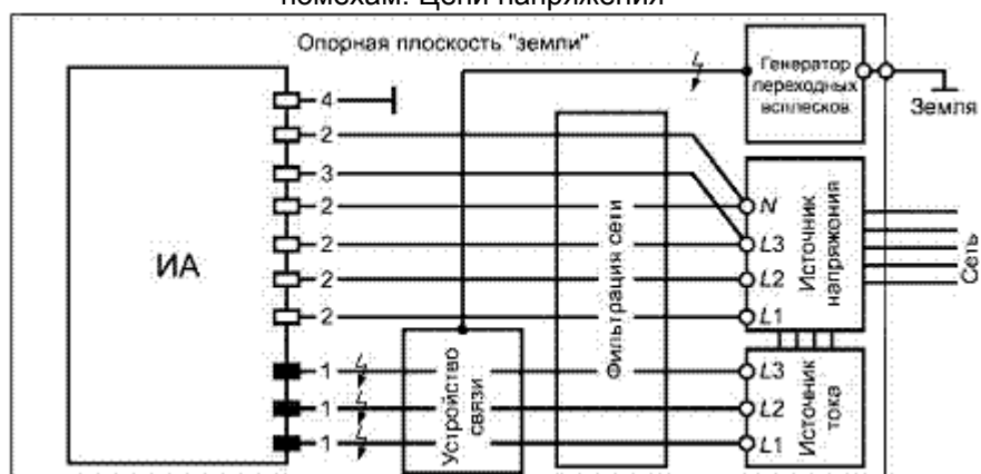
Рисунок Е.2 - Установка для проведения испытаний на устойчивость к наносекундным импульсным помехам. Цепи напряжения
