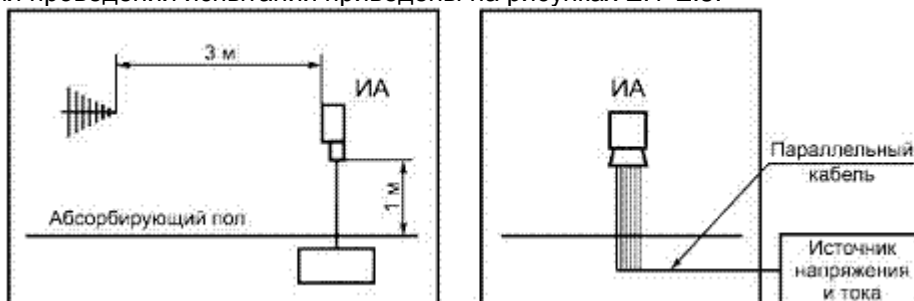
Рисунок E.1 - Установка для проведения испытаний на устойчивость к электромагнитным радиочастотным полям
