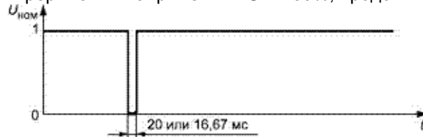
Рисунок В.2 - Прерывания напряжения \Delta U = 100\% , в течение одного цикла при номинальной частоте
