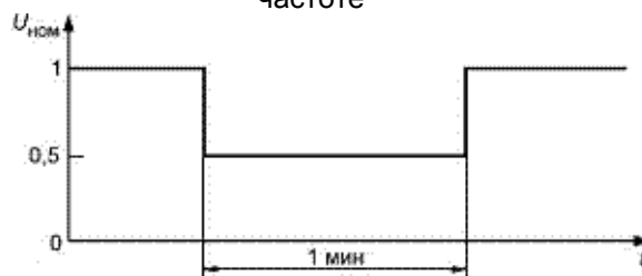
Рисунок В.3 - Провалы напряжения \Delta U = 50\%
