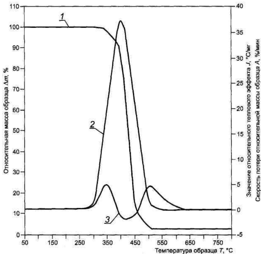
1 – ТГ-зависимость; 2 – ДТГ-зависимость; 3 – ДТА-зависимость
