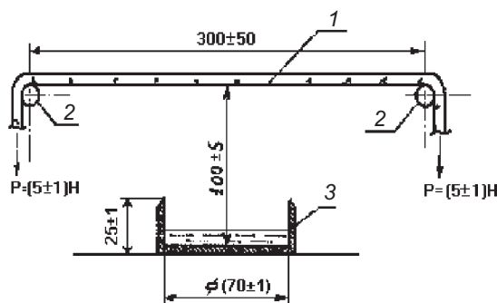
1 — образец каната (ленты); 2 — опоры; 3 — емкость для горячего
