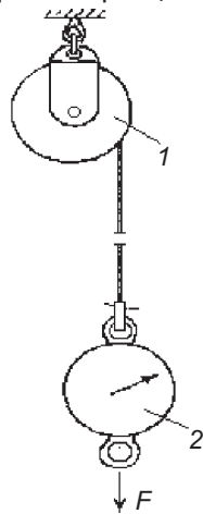
1 — УКСПа; 2 — динамометр
