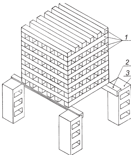
1 — деревянные бруска; 2 — стальной уголок; 3 — бетонный (металлический) блок
