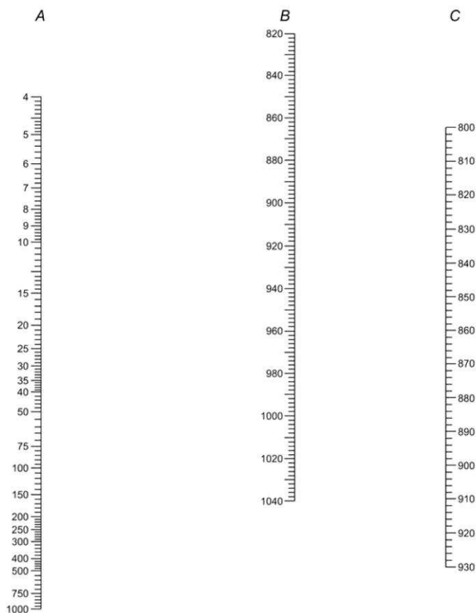
Рисунок J.1 - Номограмма для получения CCAI
