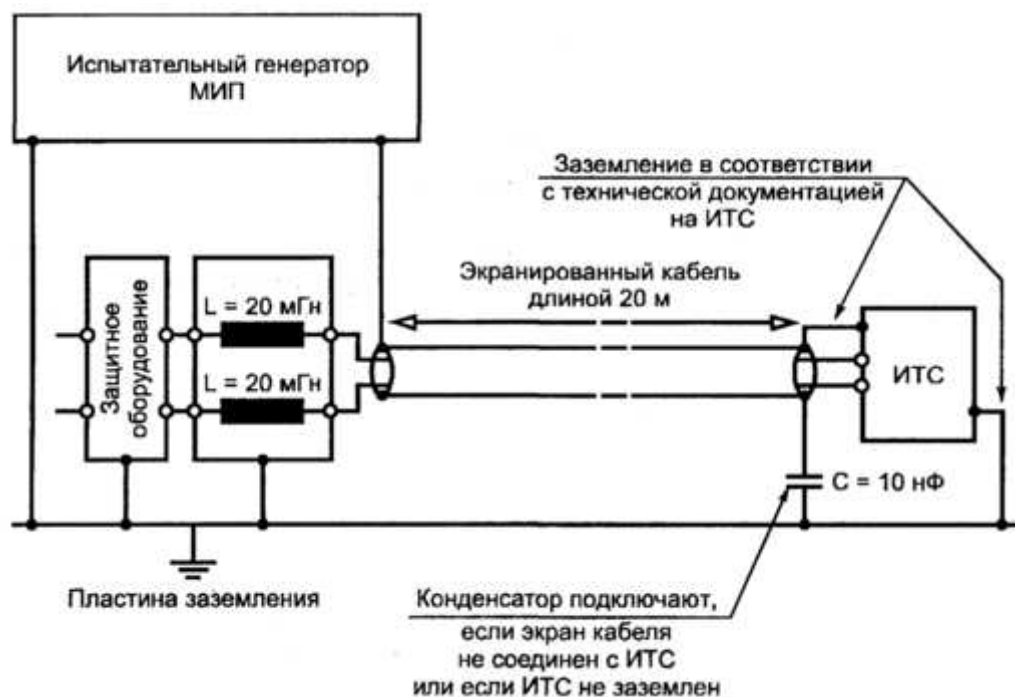
Рисунок 4 — Типичная схема ввода помех в экранированные сигнальные кабели
