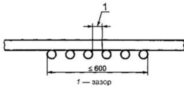
Рисунок 1 – Кабели закрепленные на передней стороне стандартной лестницы с зазором
