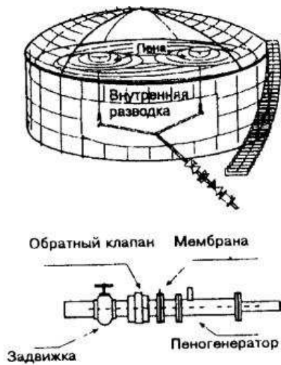
Рис. 4. Стационарная установка пожаротушения с подачей пены низкой кратности в слой горячей жидкости (подслойный способ тушения пожара)
