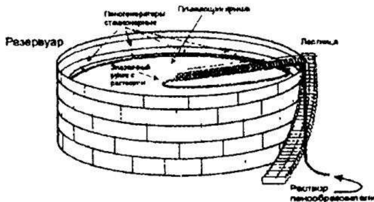
Рис. 6. Пеночамера с пеногенератором для образования и подачи пены низкой кратности в резервуар с плавающей крышей
