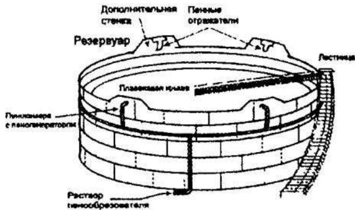
Рис. 5. Защита резервуара с плавающей крышей стационарной установкой пожаротушения с подачей пены низкой кратности
