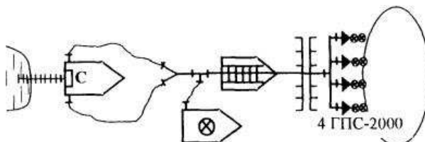
Рис. 1. Принципиальная схема тушения пожара в резервуаре пеной средней кратности с использованием механизированного пеноподъемника
