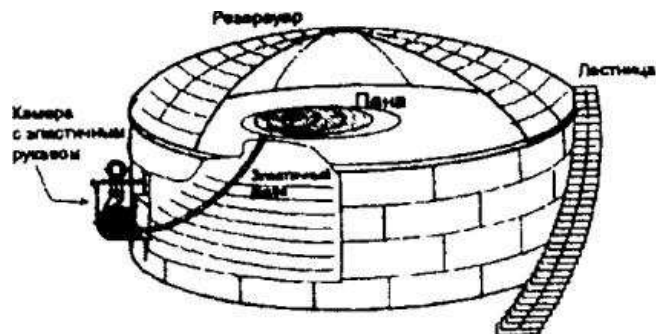
Рис. 2. Применение раздвижных пеносликов для плавной подачи пены на поверхность нефтепродукта
