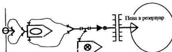
Рис. 2. Принципиальная схема подачи пены низкой кратности при тушении пожара в резервуаре подслоиным методом
