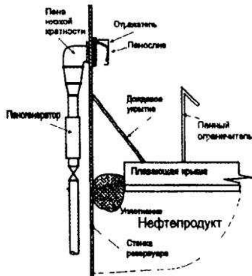
Рис. 6. Пеночамера с пеногенератором для образования и подачи пены низкой кратности в резервуар с плавающей крышей
