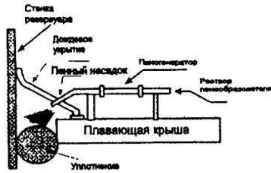
Рис. 8. Расположение пеногенерирующей аппаратуры на плавающей крыше
