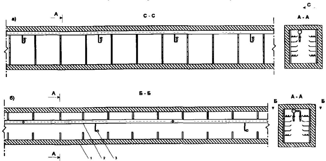
Схема установки оросителей в кабельном туннеле
