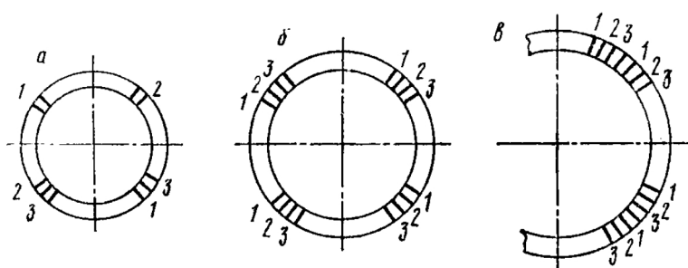
Рис. 3. Схема вырезки образцов для механических испытаний
