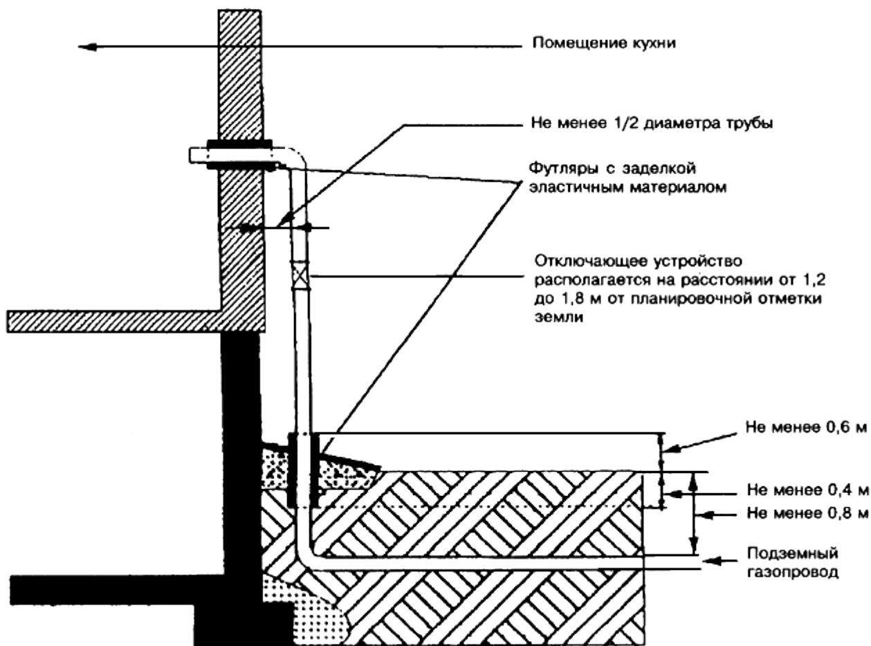
Рисунок 9.1 - Газовый ввод
