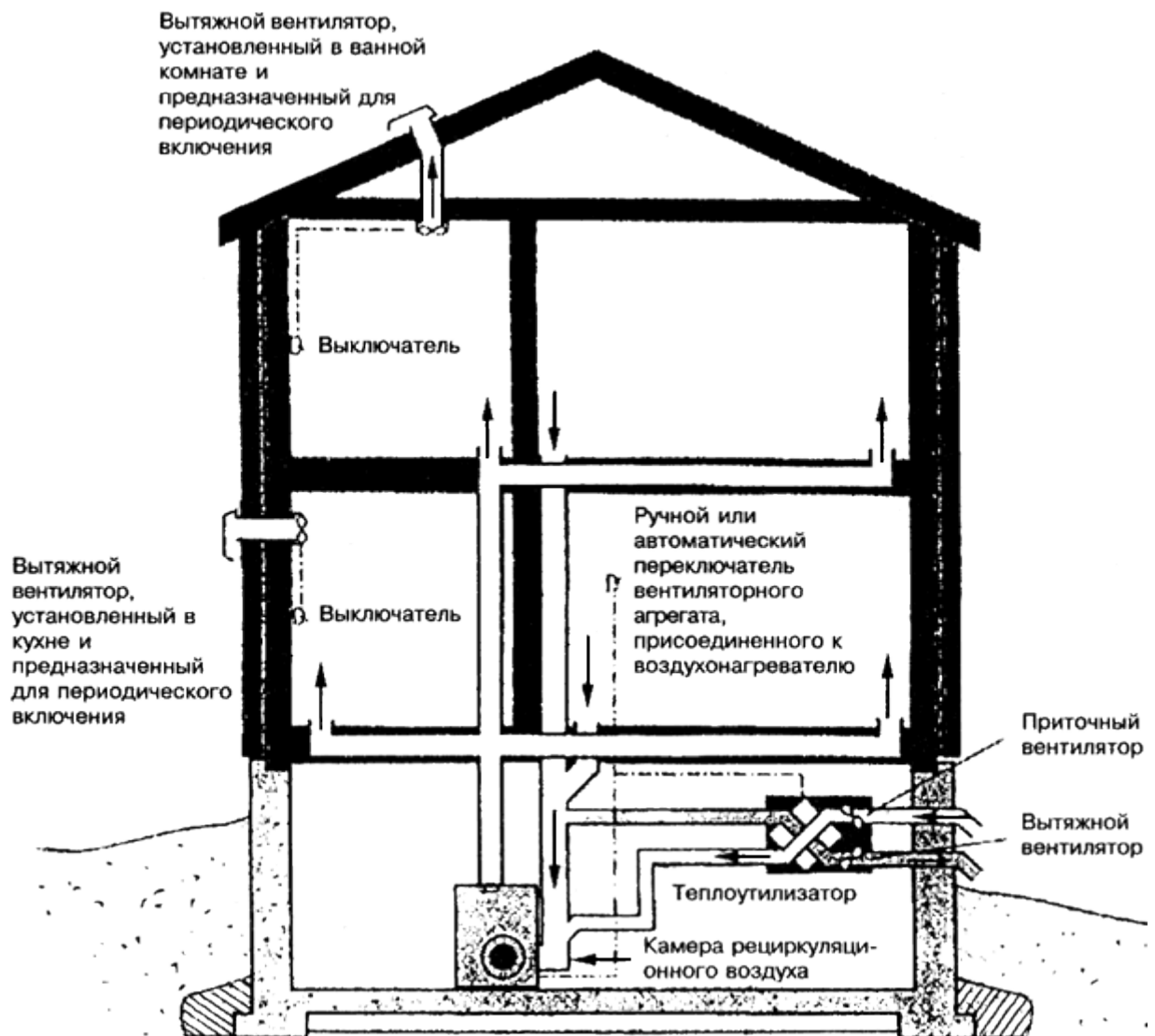
Рисунок 7.3 - Присоединение теплоутилизационного агрегата к камере подогрева воздуха
