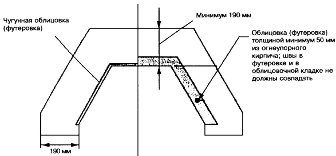
Рисунок 7.5 - Футеровка камина
