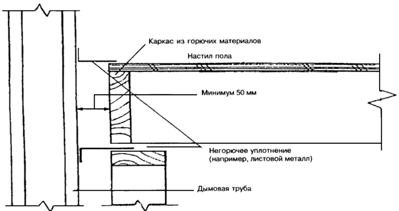
Рисунок 7.8 - Расстояние от дымовой трубы до строительных конструкций
