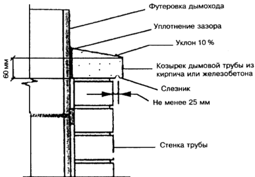
Рисунок 7.7- Оголовок дымовой трубы
