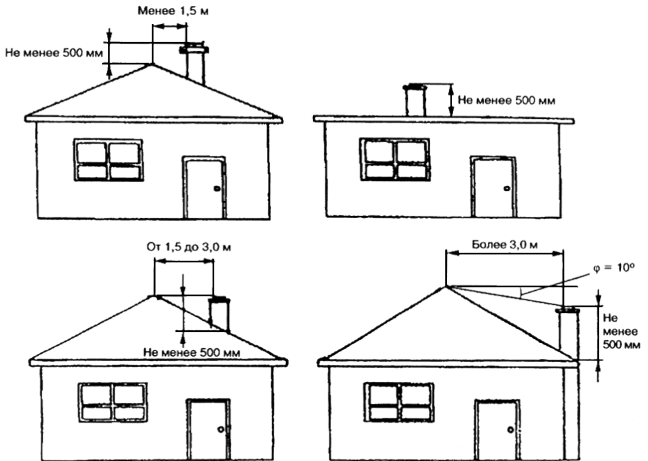
Рисунок 7.9 - Минимальная высота дымовой трубы
