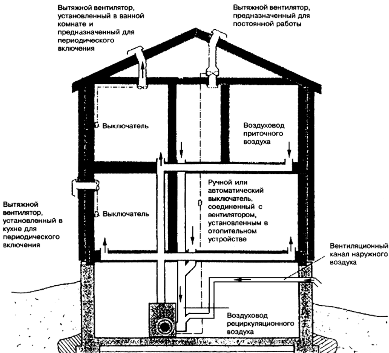
Рисунок 7.1 - Система воздушного отопления с принудительной циркуляцией воздуха, совмещенная с системой механической вентиляции, присоединенная к системе теплоснабжения
