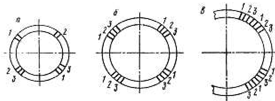
Рис.3 - Схема вырезки образцов для механических испытаний
