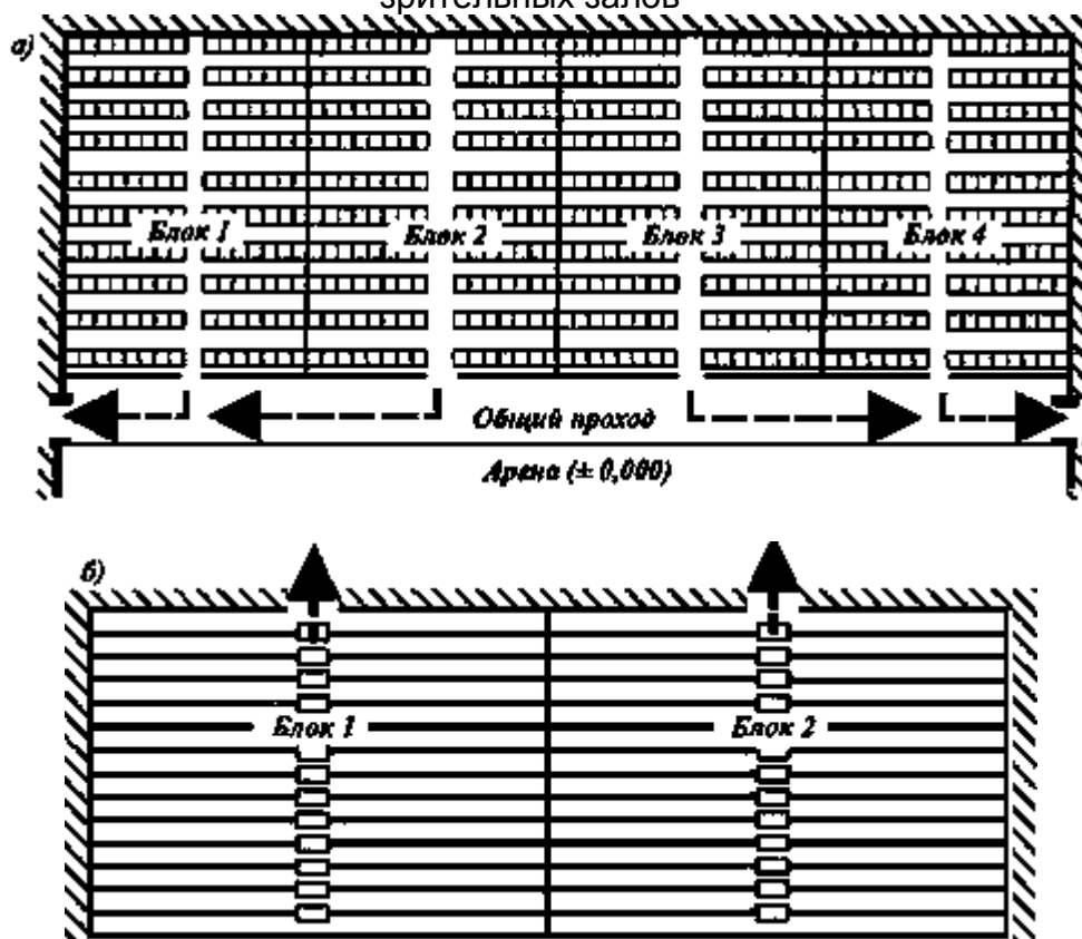
а - при эвакуации в общий горизонтальный проход на уровне арены; б - при эвакуации вверх через дверной проем или на горизонтальный участок Рисунок И.2 - Схемы разделения мест на блоки на трибунах спортивно-зрелищных и универсальных залов при расположении люков
