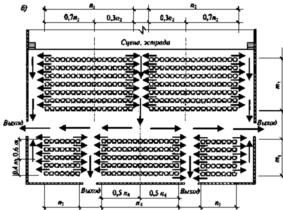
а - с боковыми (продольными) проходами; б - с поперечным проходом Рисунок И.1 - Маршрутизация движения людских потоков при эвакуации из зрительных залов
