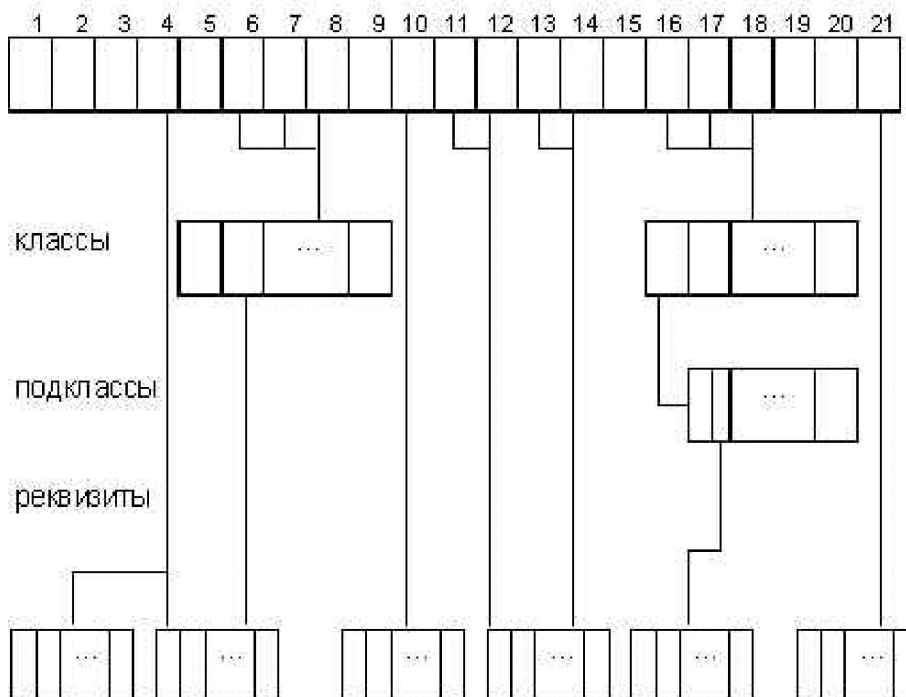
Рис.2. Структура классификатора.
