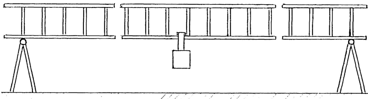
Рис. 2 Испытание лестницы, установленной на ребро, на прочность.
