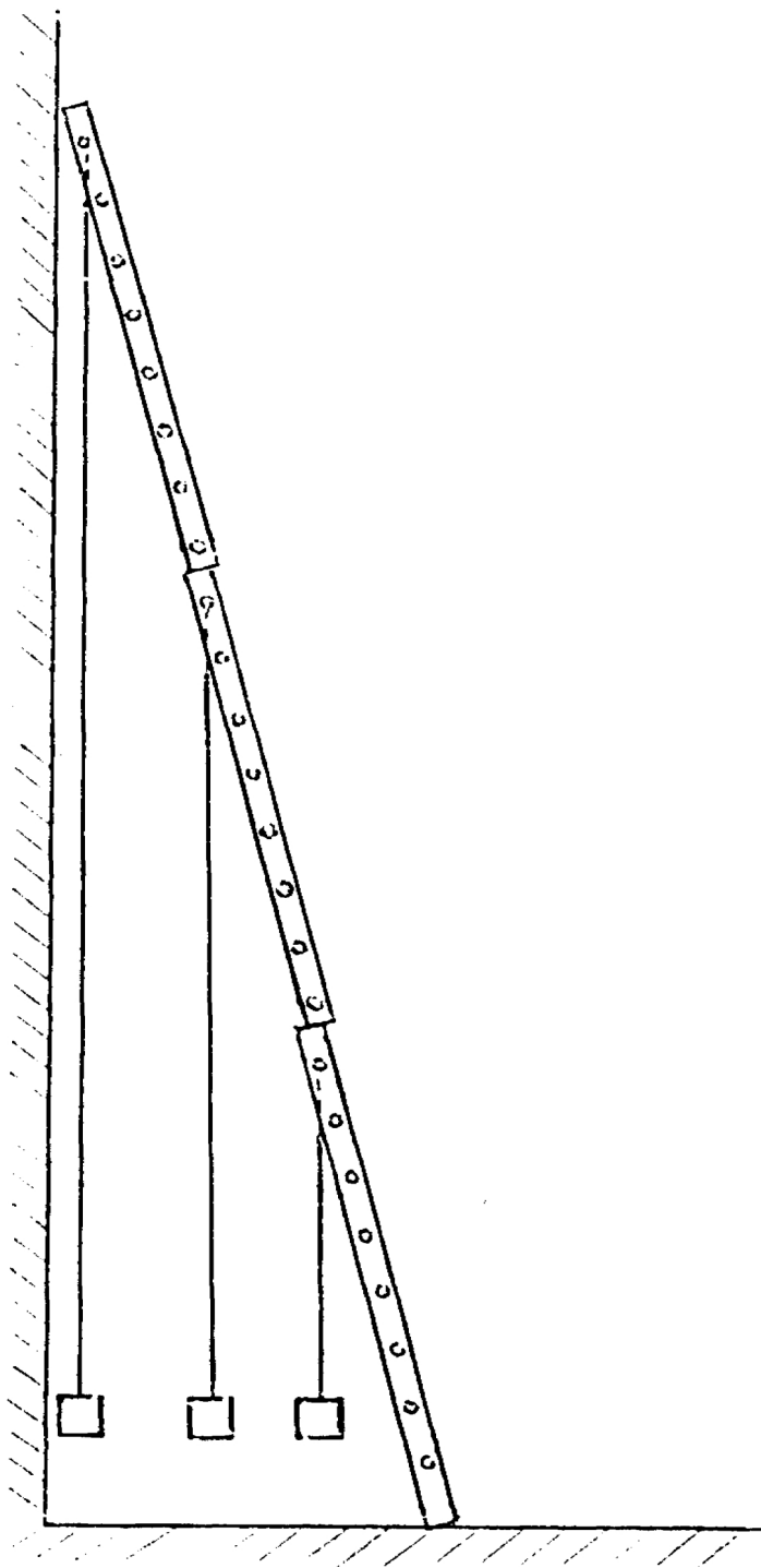
Рис. 13. Испытание выдвижной лестницы в рабочем положении на прочность.
