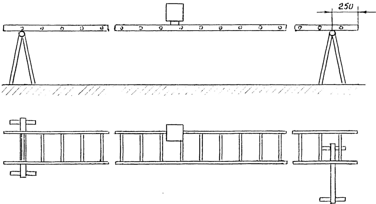
Рис. 3 Испытание лестницы на кручение.
