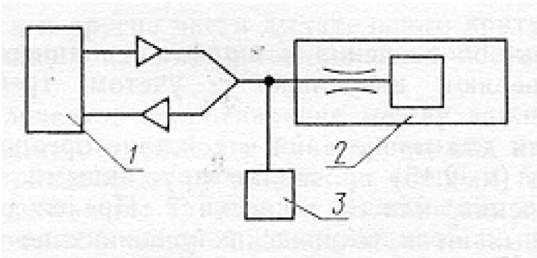
Рисунок 3. Схема проверки максимального рабочего давления в дыхательном контуре
