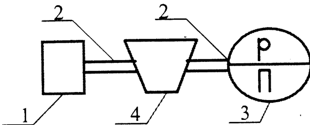
Рисунок 4. Схема проверки максимального вакуумметрического давления при аспирации
