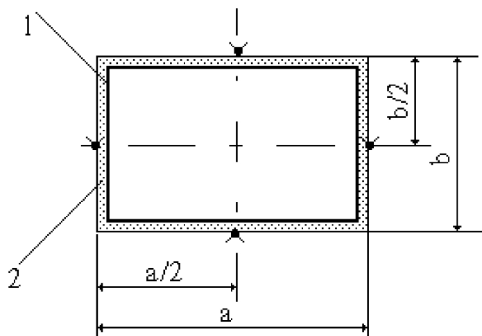
Рис. 1.4. Схема размещения ТЭП на необогреваемой поверхности воздуховода.
