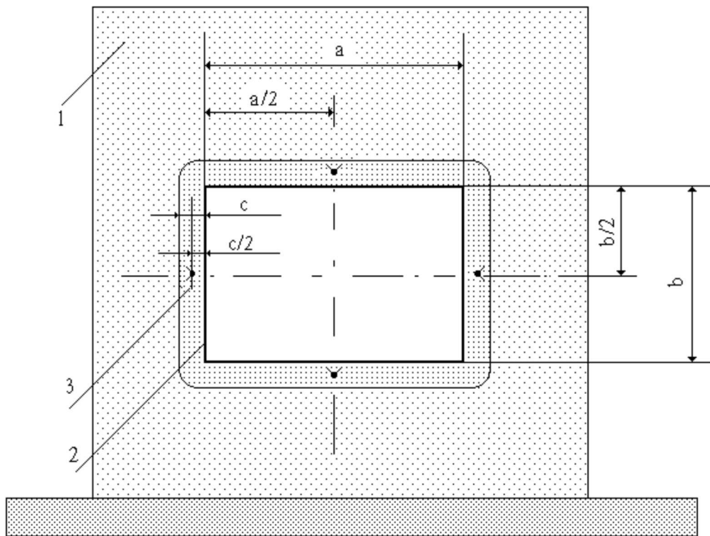
1 - печь; 2 - воздуховод; 3 - уплотнение места проходки воздуховода через ограждающую конструкцию печи; \nabla - ТЭП; a , b - внутренние размеры поперечного сечения воздуховода; c - толщина заделки
