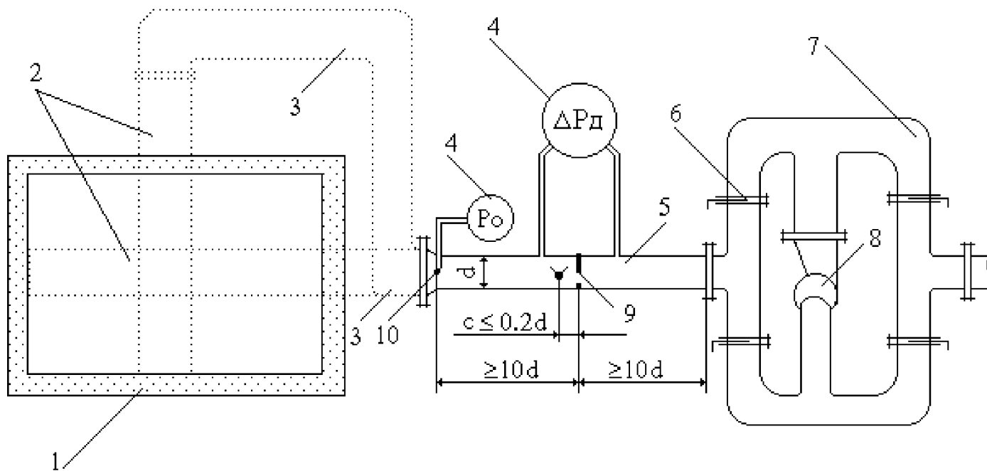
1 - печь; 2 - испытываемый образец воздуховода (установленный вертикально или горизонтально); 3 - переходной элемент; 4 - микроманометр; 5 - мерный участок; 6 - регулирующая заслонка; 7 - воздуховоды обвязки вентилятора; 8 - вентилятор; 9 - расходомерная диафрагма; 10 - точка отбора давления в полости испытываемого образца; ▼ - ТЭП
