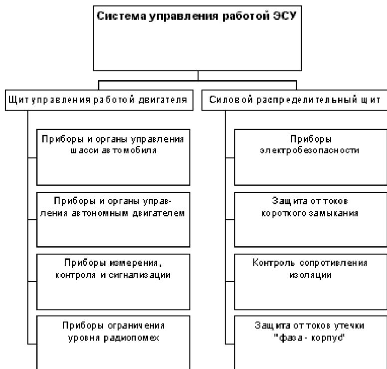
Структура системы управления работой ЭСУ АСА
